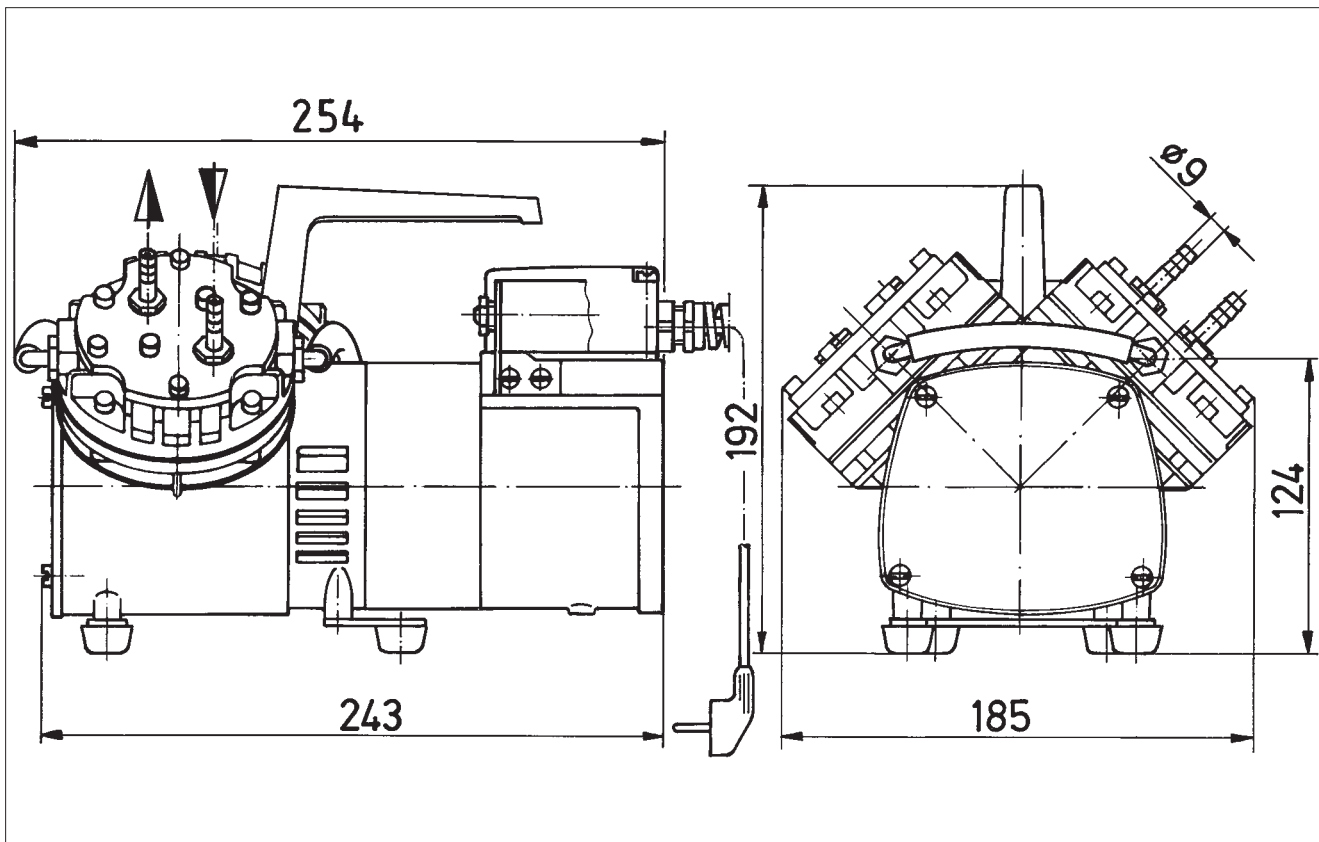
Maße (mm)
